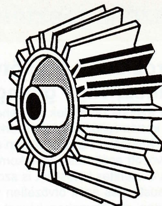
Fogaskerék törött fogának felrakása OK 68.82 elektródával.
