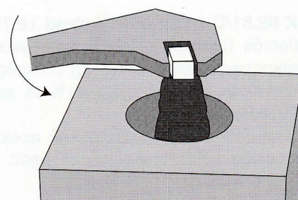
Törött csavar maradékának eltávolítása OK 68. 82 elektródával.
