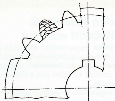
Fogaskerék törött fogának felrakása OK 68.82 elektródával.
