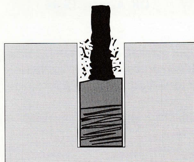
Törött csavar maradékának eltávolítása OK 68. 82 elektródával.
